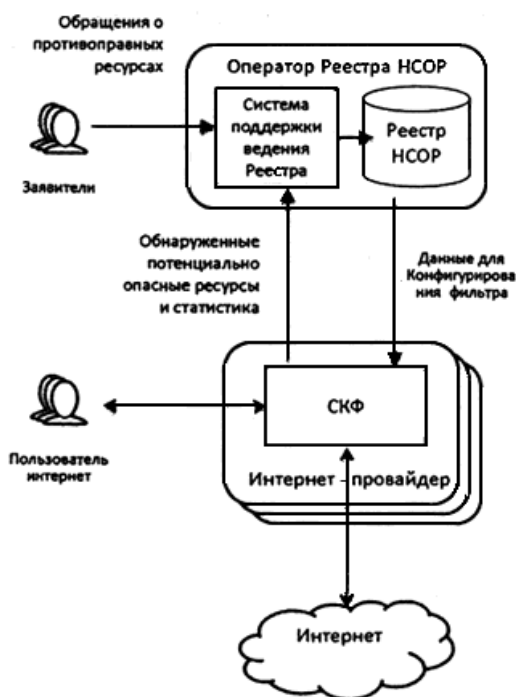
Рис. 6. Принцип контроля доступа через Реестр НСОР
